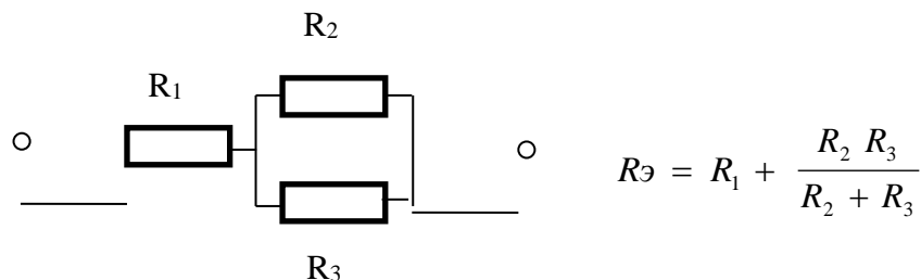
Рисунок 5 – Схемы соединений
